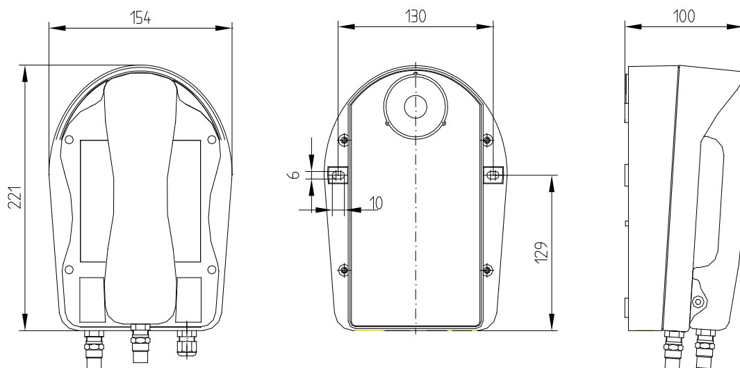
Abbildung 1: Maßzeichnung 1 DAH 02
