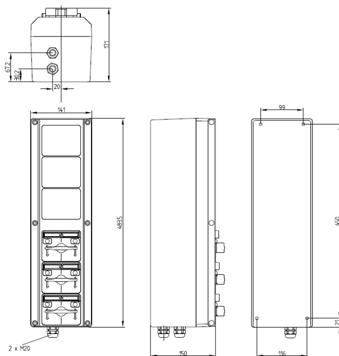
Abbildung 1: Maßzeichnung 6/12 DAZ 005
