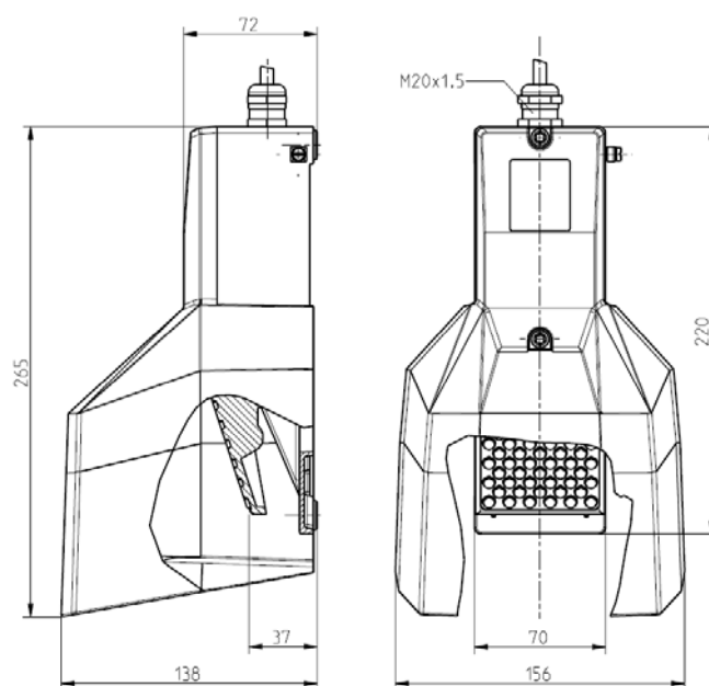
Abbildung 1: Maßzeichnung 1 FSX 21
