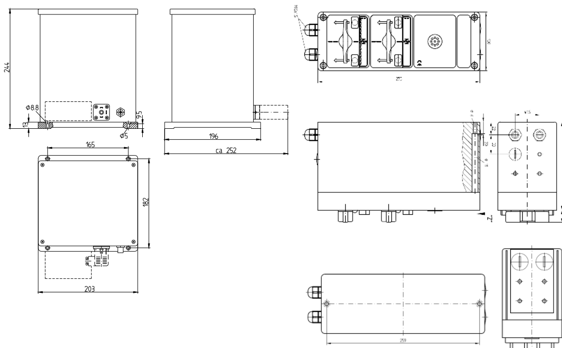
Abbildung: Maßzeichnung 4 FKUD .. bzw. 4 FKVD ..
