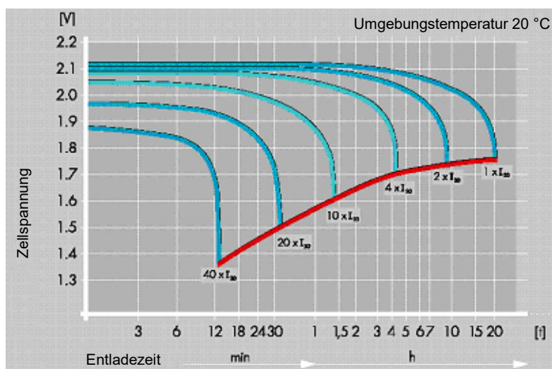
Abb. 1: Entladedaten 4 NSV
