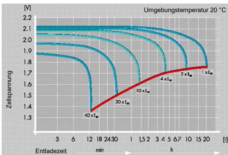
Abb. 1: Entladedaten 5 NSV
