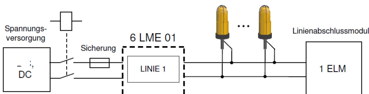
Beispiel 2: Blitzlampenüberwachung
