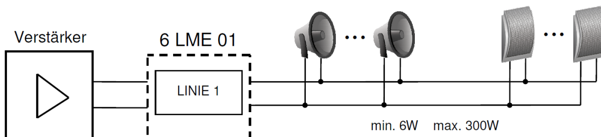
Beispiel 1: Lautsprecherüberwachung
