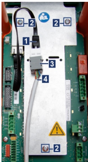
Abb. 14: NRO 0x2 mit einer Ethernet-Schnittstelle
