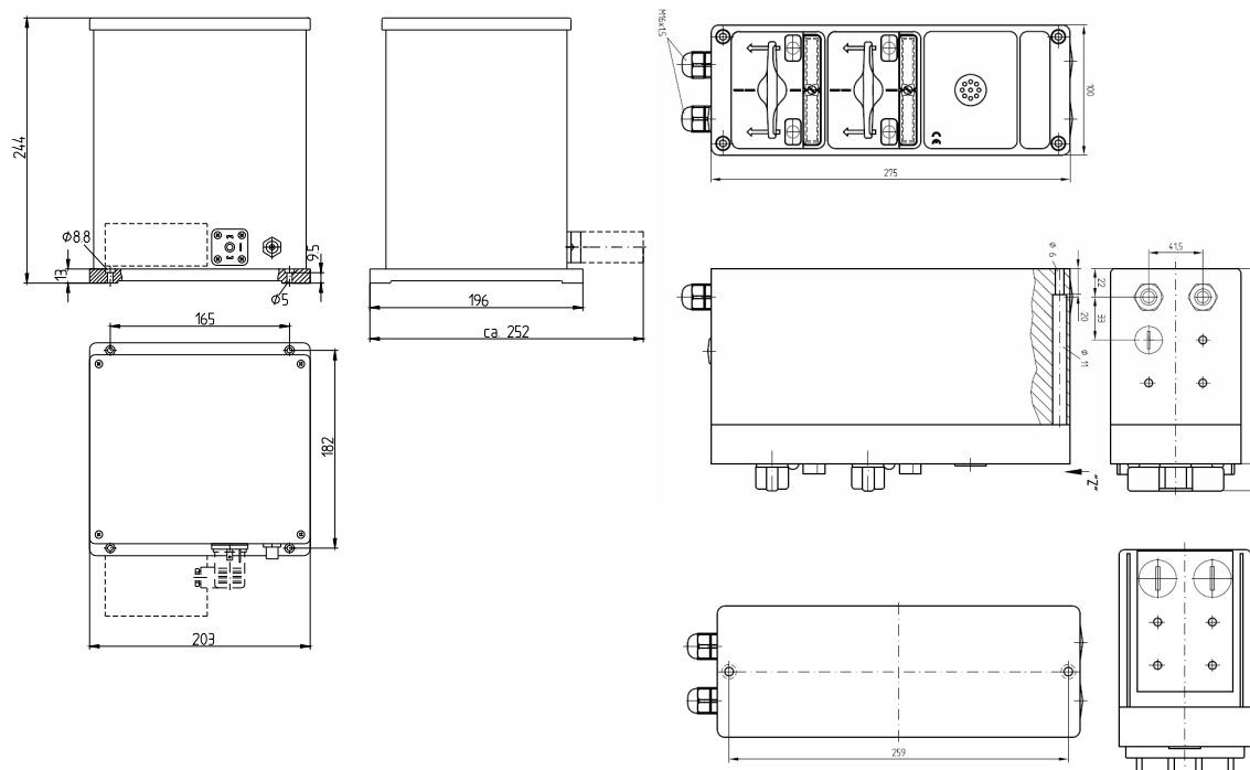
Abbildung: Maßzeichnung 4 FKUH 10 bzw. 4 FKVH 10
