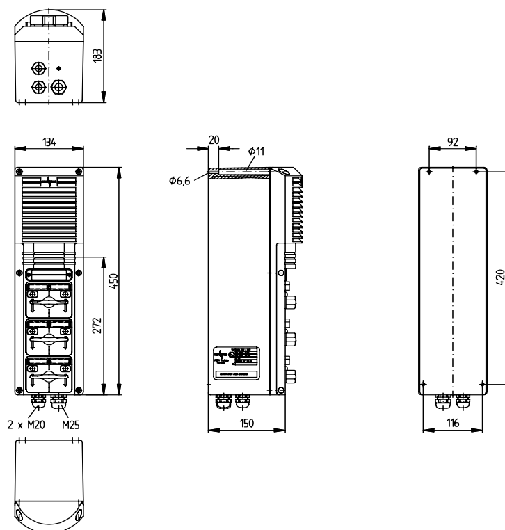
Abbildung 1: Maßzeichnung DA 004
